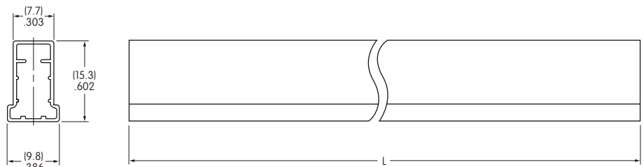
Stick-Tube Dimensions
